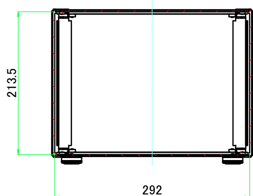
A-A ( 1 : 5.5 )
